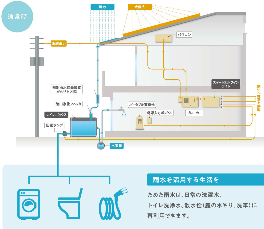
図2 「GQ システム Light-Plus」イメージ図 (平常時)
